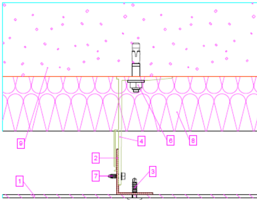
Figure 8 – Ossature intermédiaire
