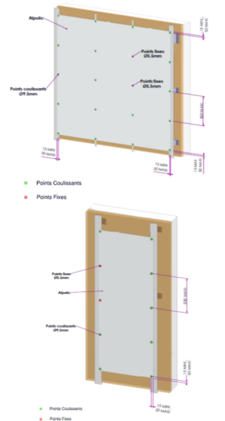
Figure 1bis – Points fixes et points de dilatation
