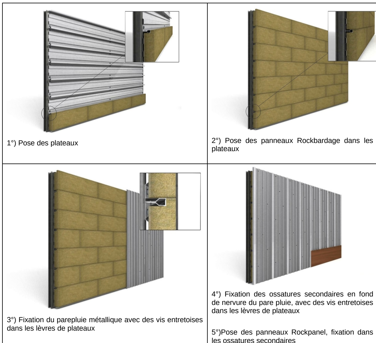
Figure 25 – Séquentiel de pose avec pare-pluie métallique
