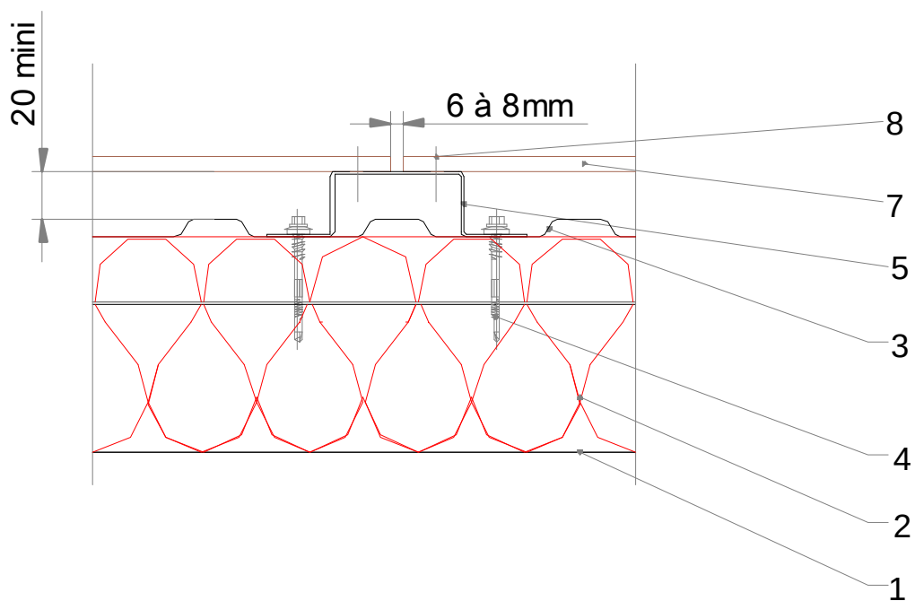
Figure 7 – Jonction entre panneaux – Coupe horizontale
