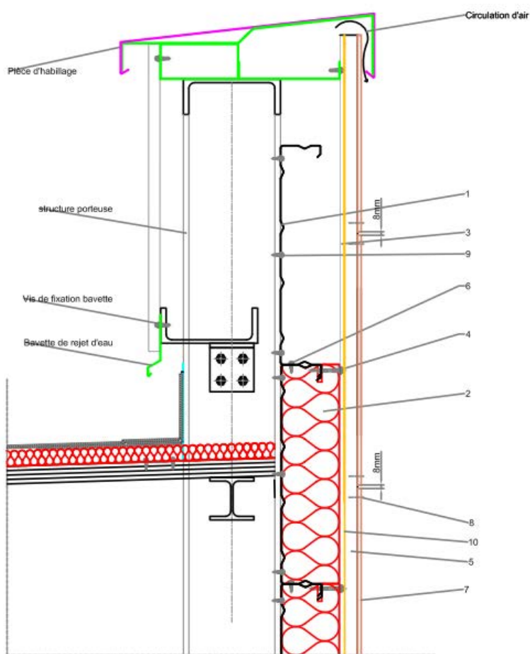
Figure 9 – Arrêt sur acrotère – Coupe verticale
