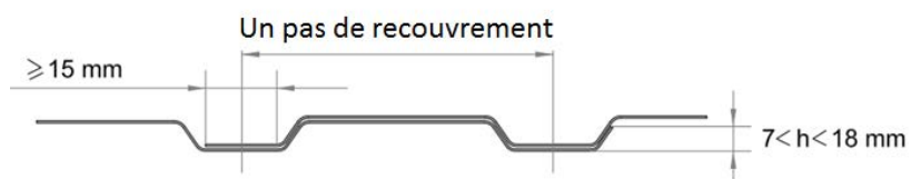
Figure 10bis – Recouvrement minimal du pare pluie métallique lorsque la hauteur des nervures est inférieure à 15mm
