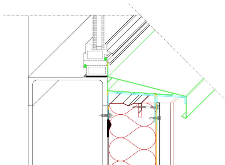
Figure 17 – Appui de baie – Coupe verticale
