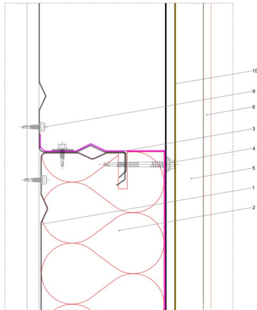
Figure 9quater – Détail sur fixation pare pluie synthétique
