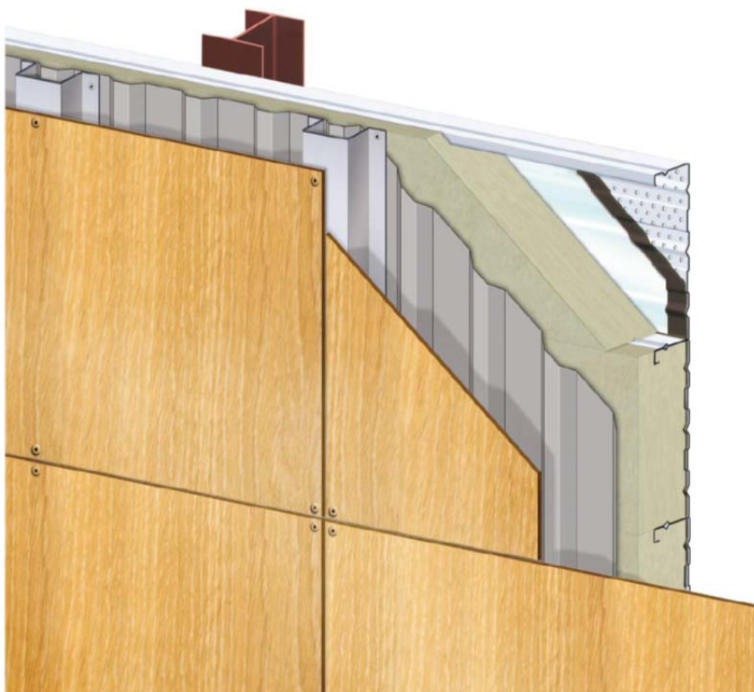
Figure 1 – Schéma de principe avec pare-pluie métallique
