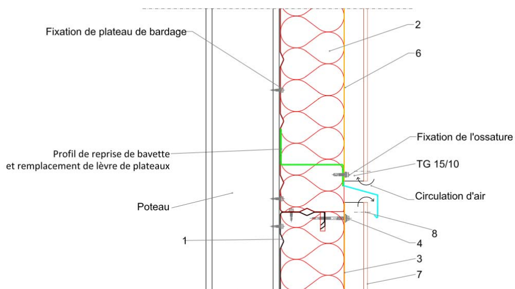
Figure 27 – Recouplement du pare-pluie souple tous les 6m
