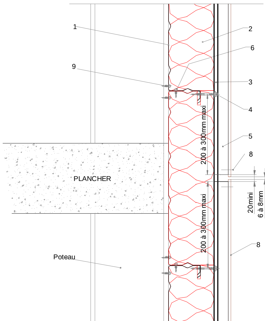
Figure 13 – Fractionnement d'ossature – Coupe verticale
