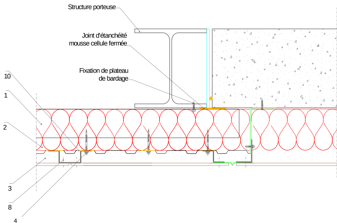
Figure 21 – Jonction sur maçonnerie
