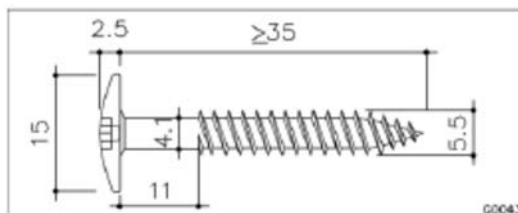
Figure 3 - Vis UNIVIS Ø 5,5 x 35mm pour plaques EQUITONE [natura] [pictura] [textura]
