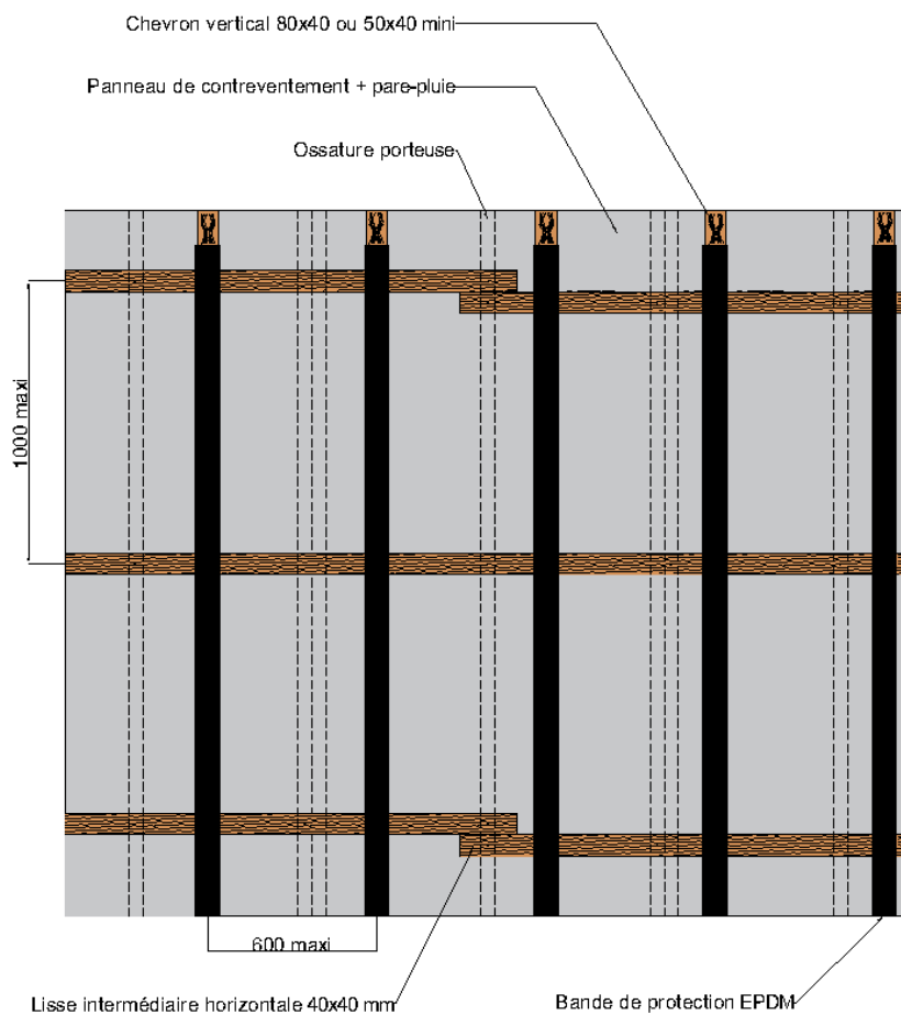
Sections minimales des chevrons verticaux
