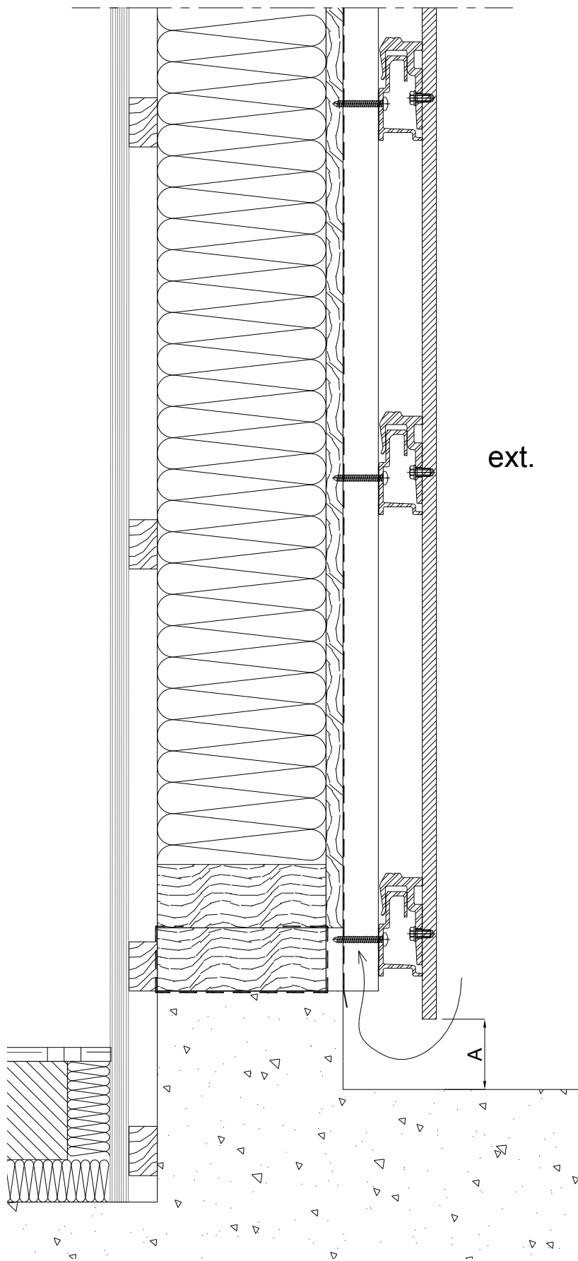
Figure 29 – Coupe verticale sur COB
