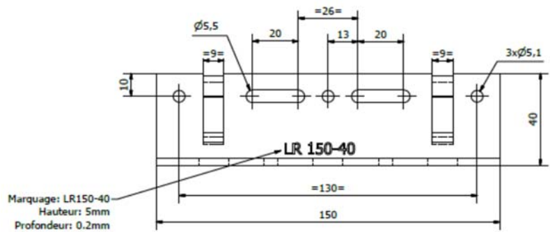
Patte-équerre ISOLALU LR 150 ETANCO
